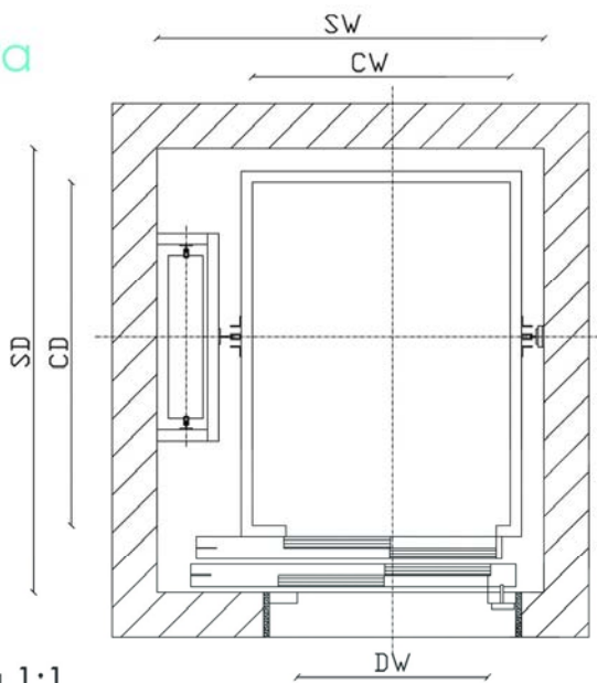
Підвіска 1:1
